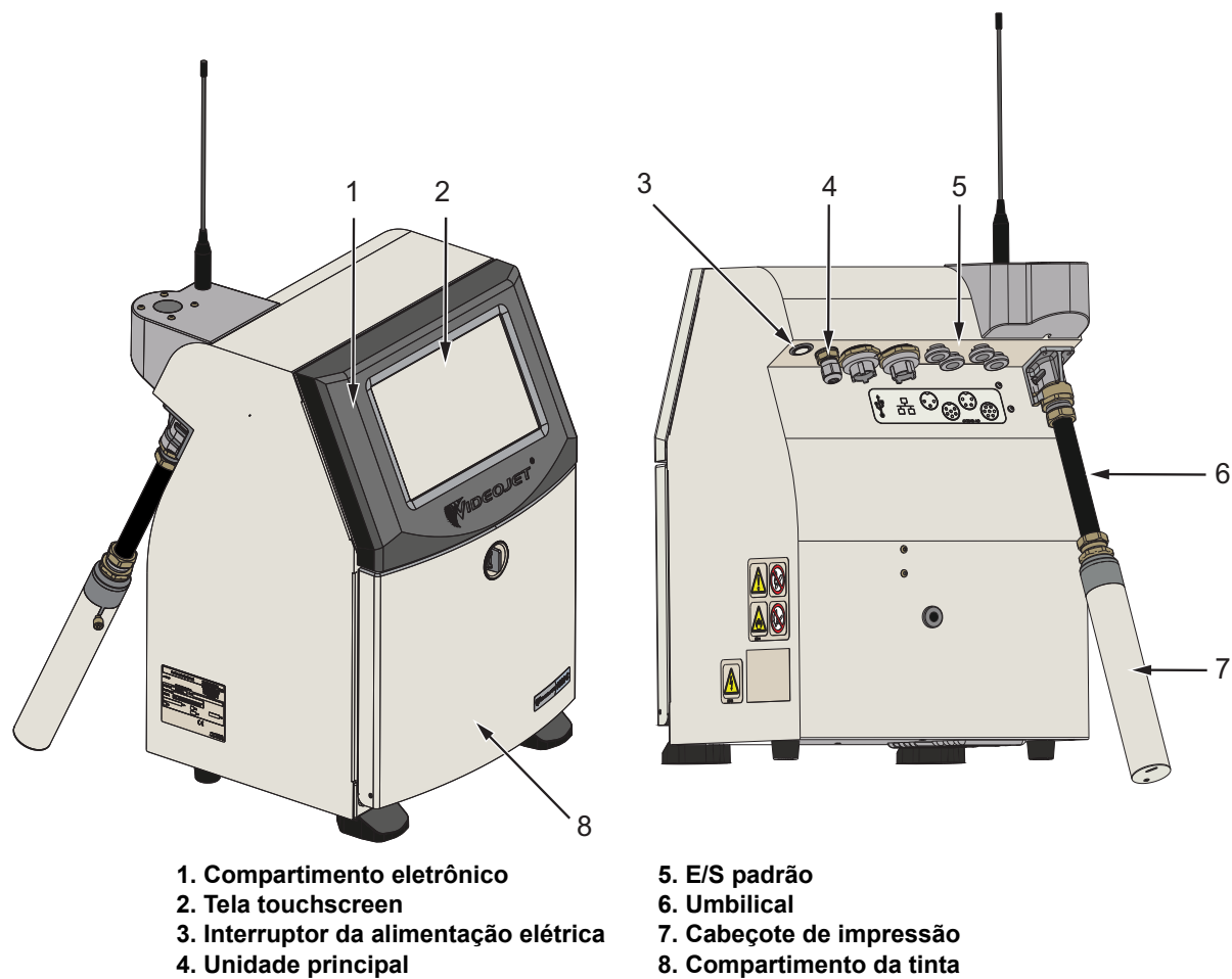
Figura 3-2: Impressora Videojet 1580 C
