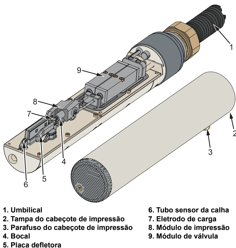
Figura 3-14: Visão geral do cabeçote de impressão
