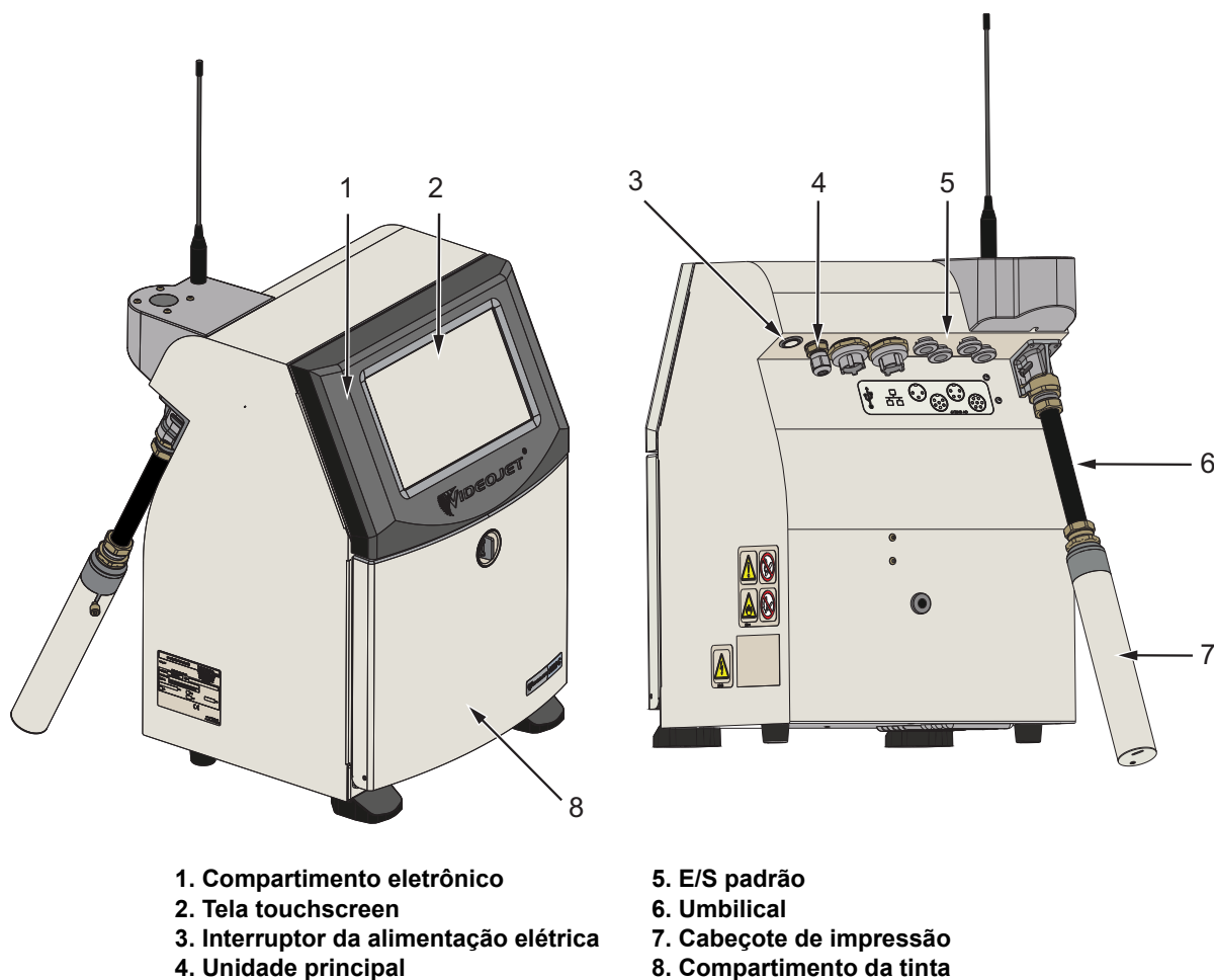
Figura 1-1: Impressora Videojet 1580 C
