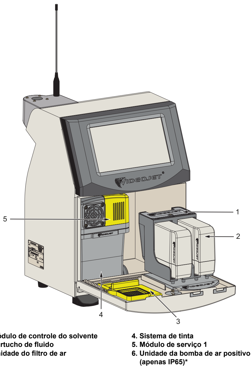
Figura 3-6: Compartimento da tinta
