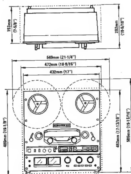
Fig. 1-1 Dimensions
