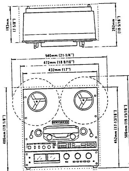
Fig. 1-1 Dimensions
