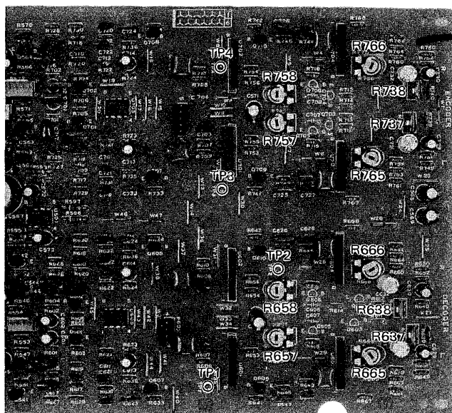
Fig. 3-16 DBX PCB
