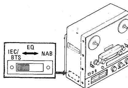
図8 NAB-BTSイコライザの切換
