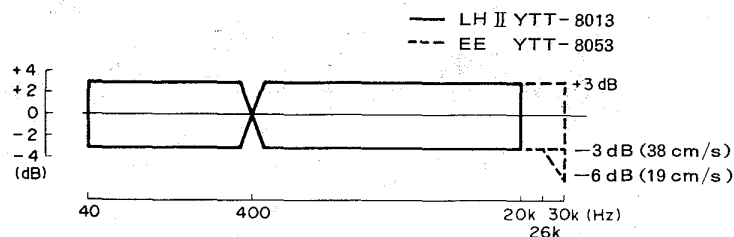
図20 録再生周波数特性 (38 cm/s, 19 cm/s)
