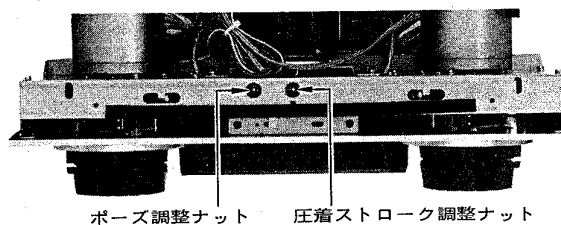
図2 ポーズ位置及び圧着ストローク調整箇所
