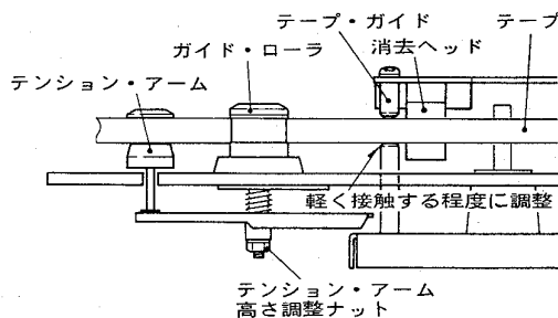
図16 テンション・アーム高さ調整
