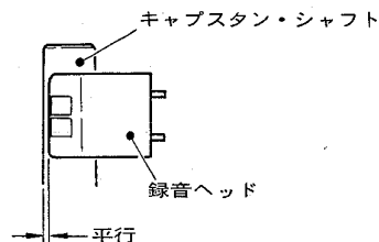
図15 録音ヘッドのあおり調整
