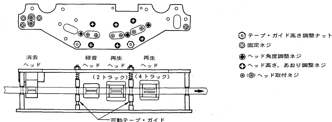
図9 テープ・ガイド及びヘッドの配列
