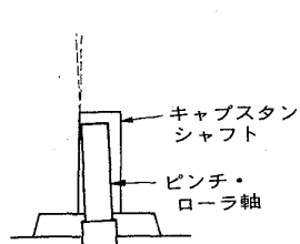
図12 B視図(平行でない例)
