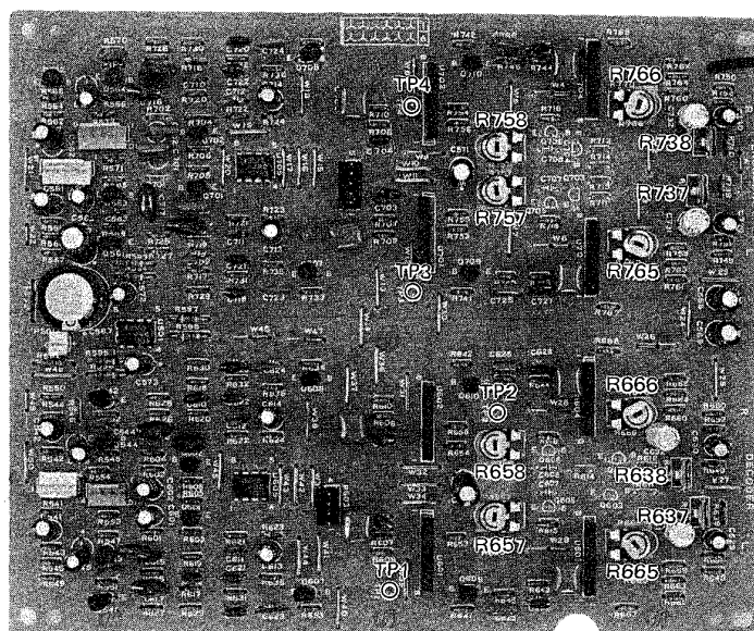
図 19 DBX 基板調整個所
