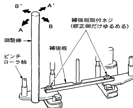
図13 ピンチ・ローラ軸傾きの修正
