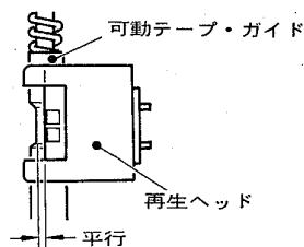
図14 再生ヘッドのあおり調整
