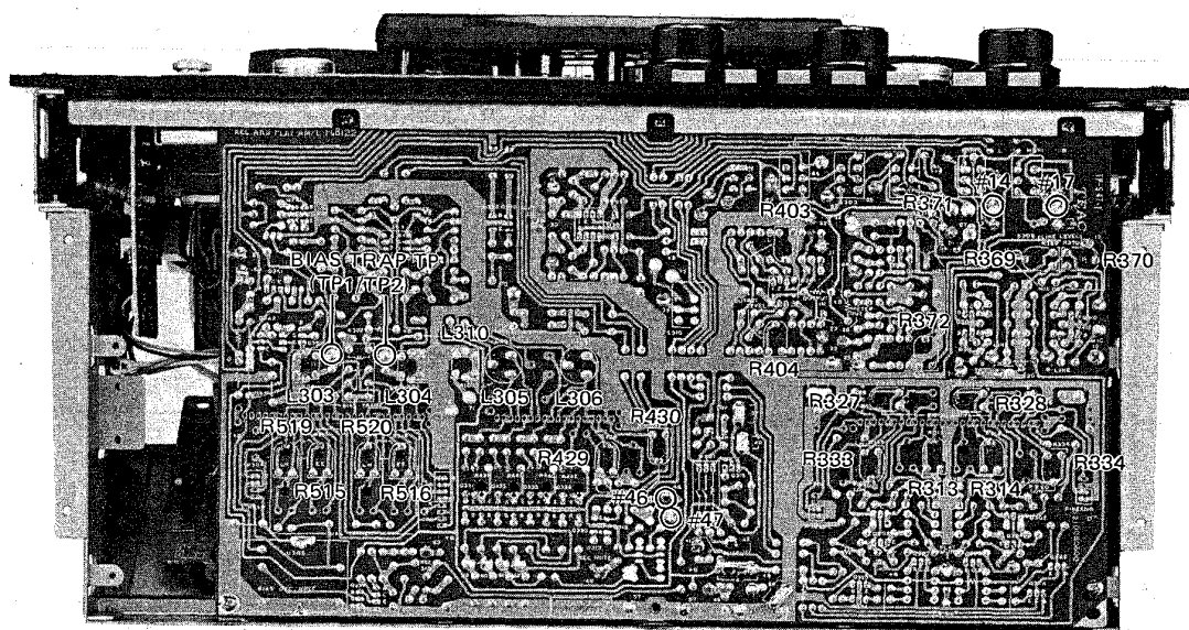
図 18 録・再基板調整個所
