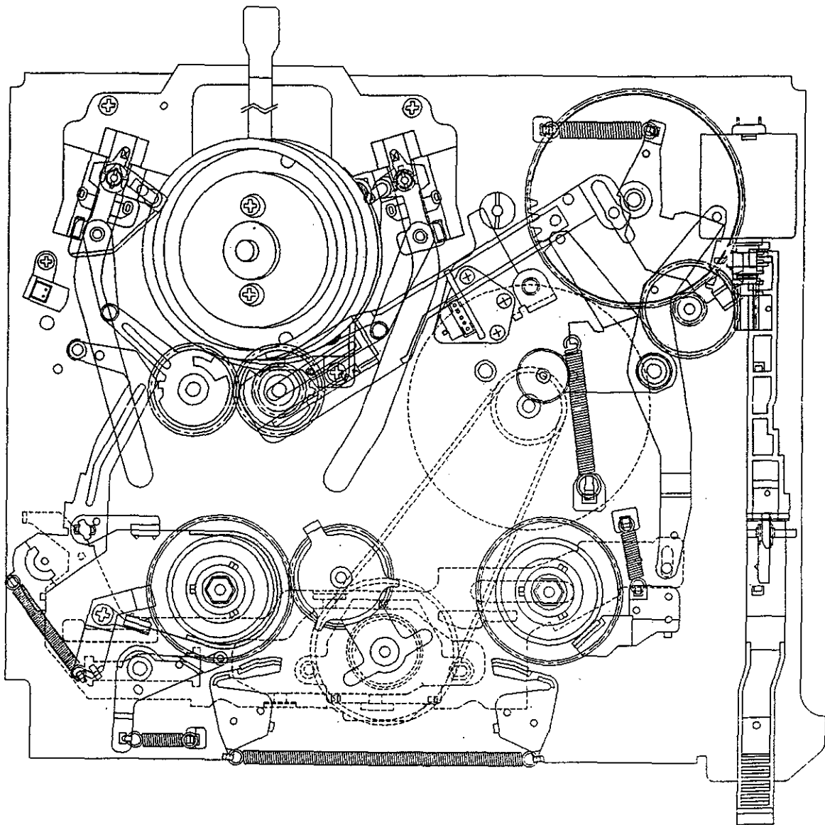
Fig. 1-4. REVIEW MODE
