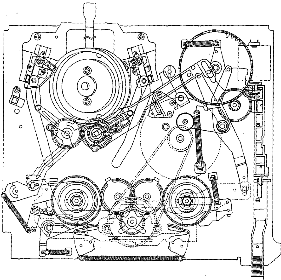
Fig. 1-9. FF/REW MODE
