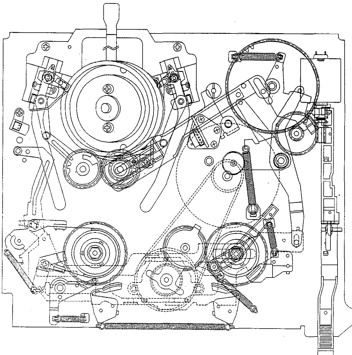
Fig. 1-7. SLOW MODE
