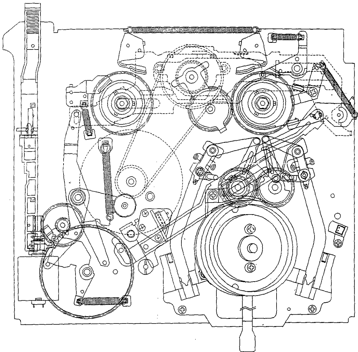
Fig. 1-2. INITIAL MODE
