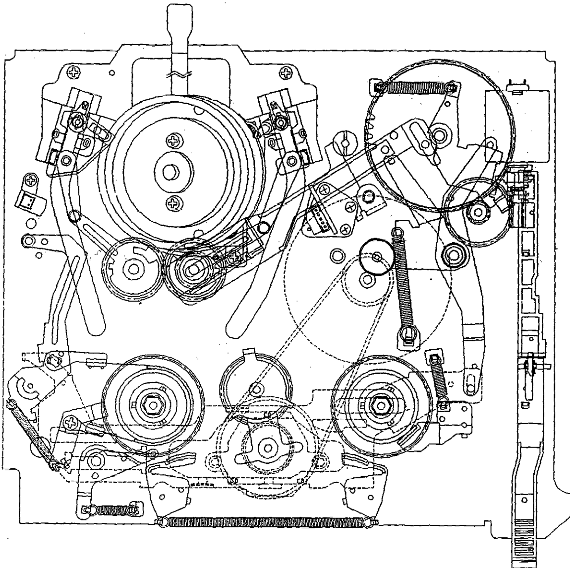
Fig. 1-5. STOP MODE
