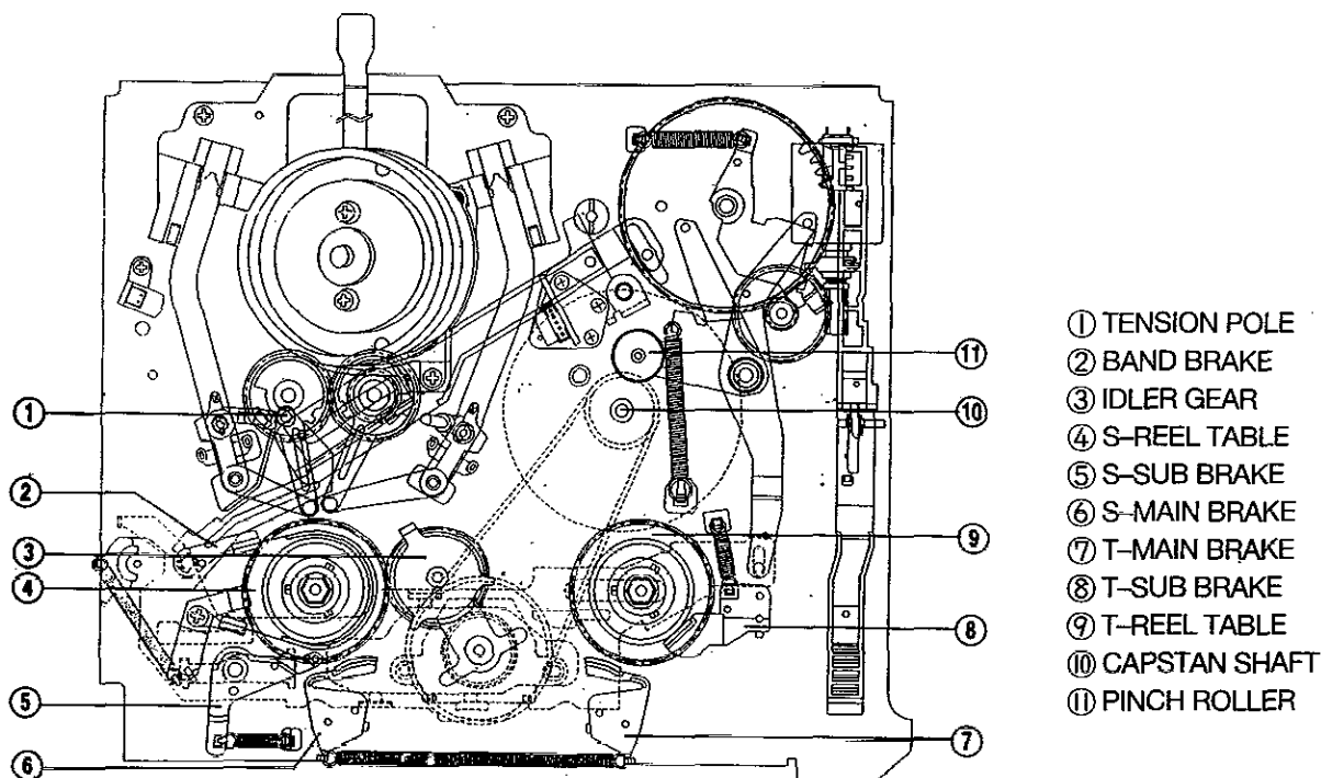
Fig. 1-1. EJECT MODE
