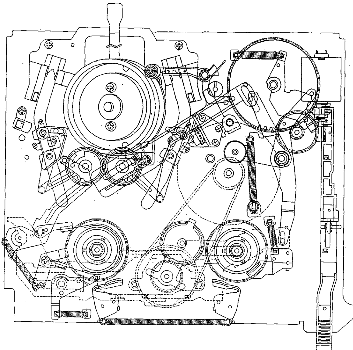
Fig. 1-3. LOADING MODE
