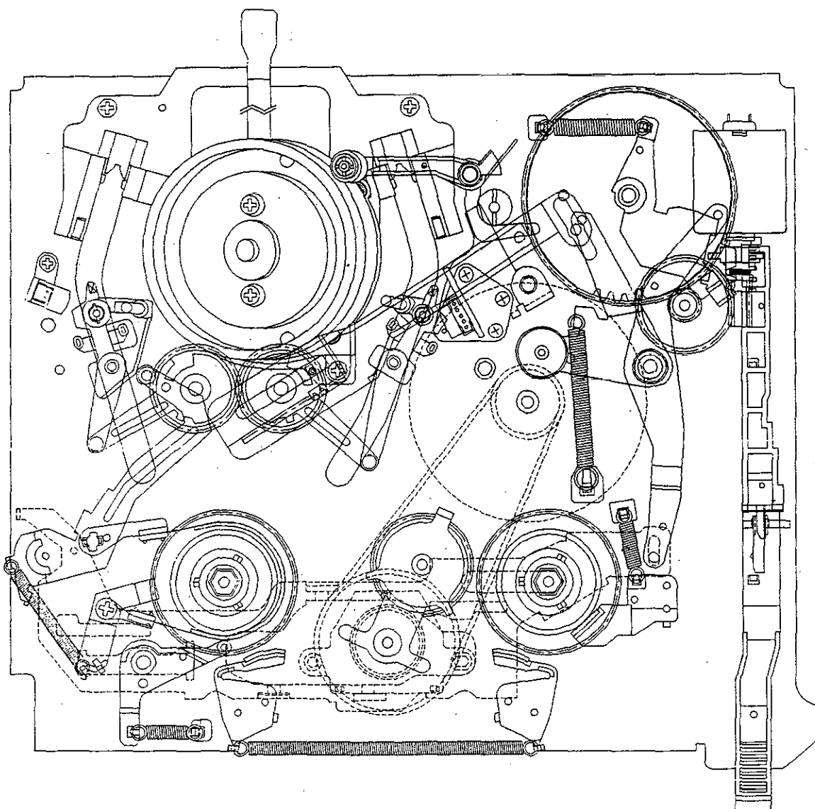
Fig. 1-3. LOADING MODE
