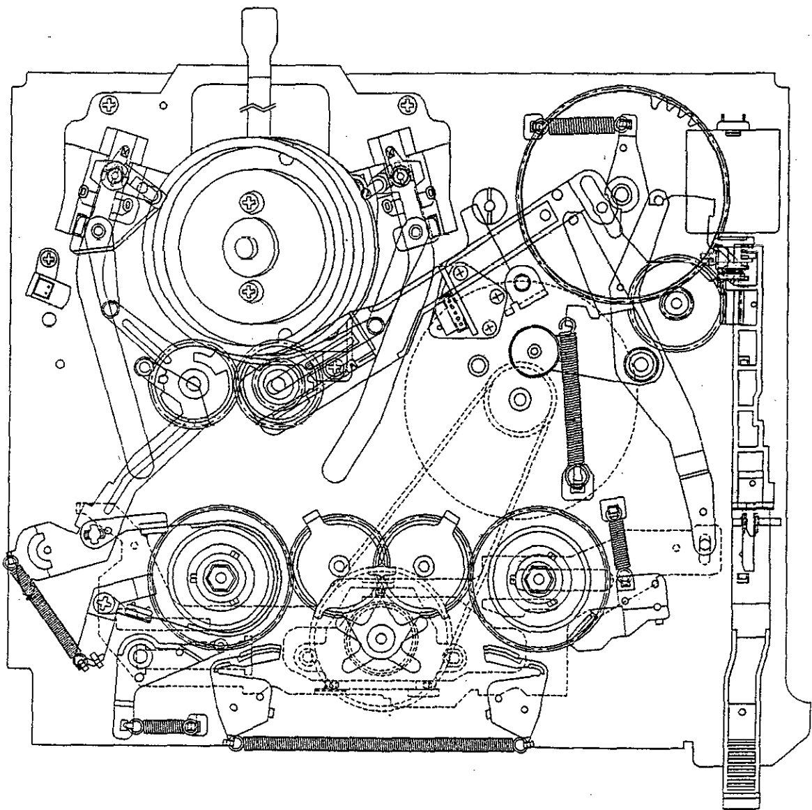
Fig. 1-9. FF/REW MODE
