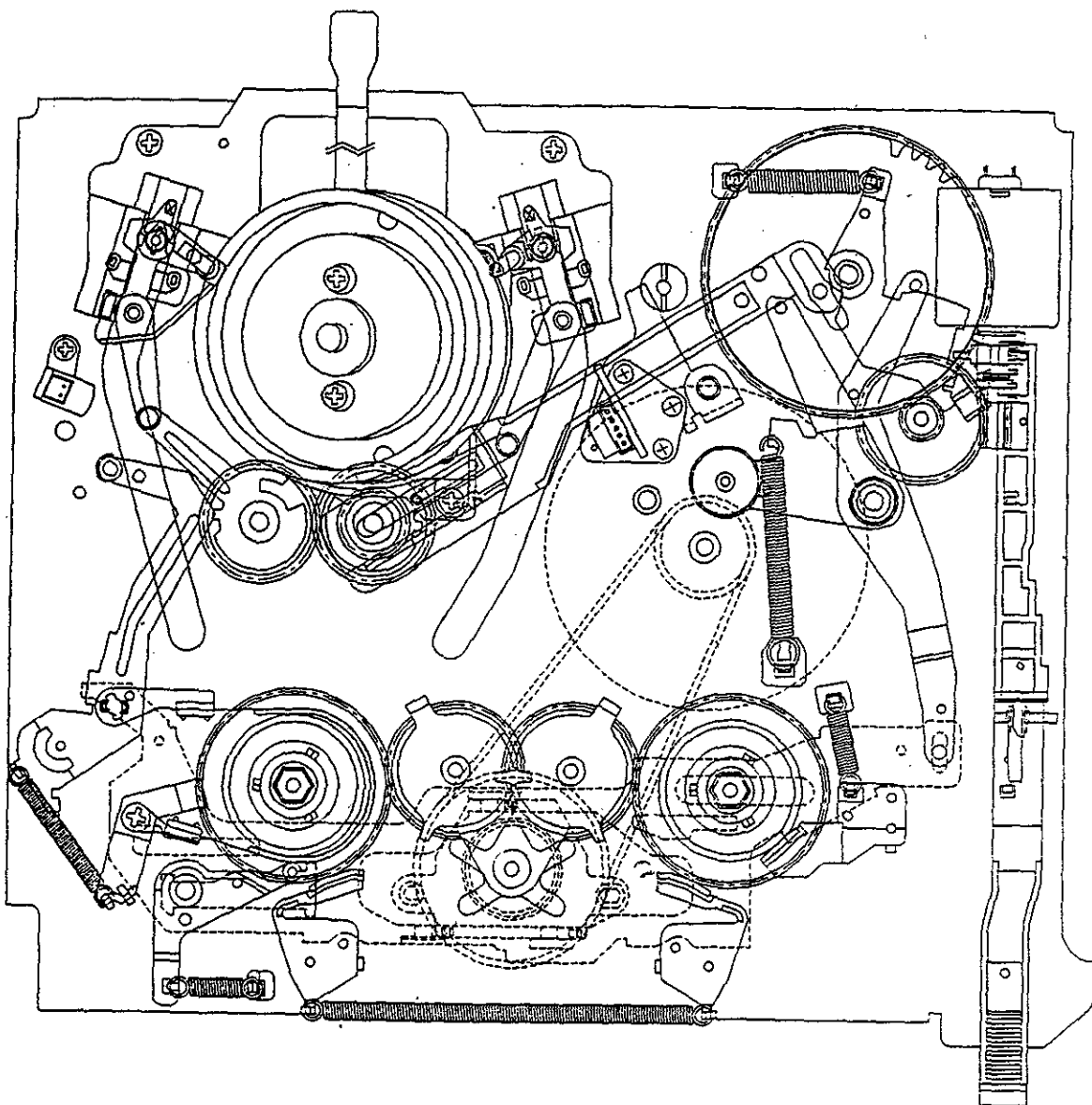
Fig. 1-8. BRAKE MODE
