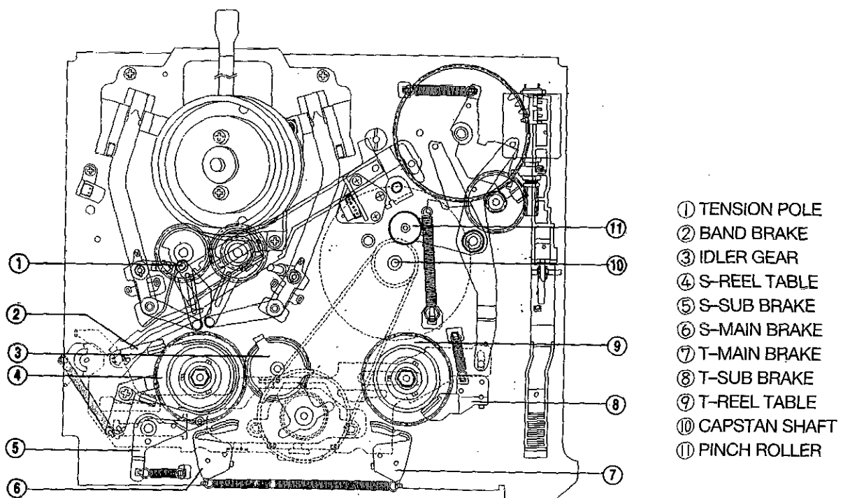
Fig. 1-1. EJECT MODE
