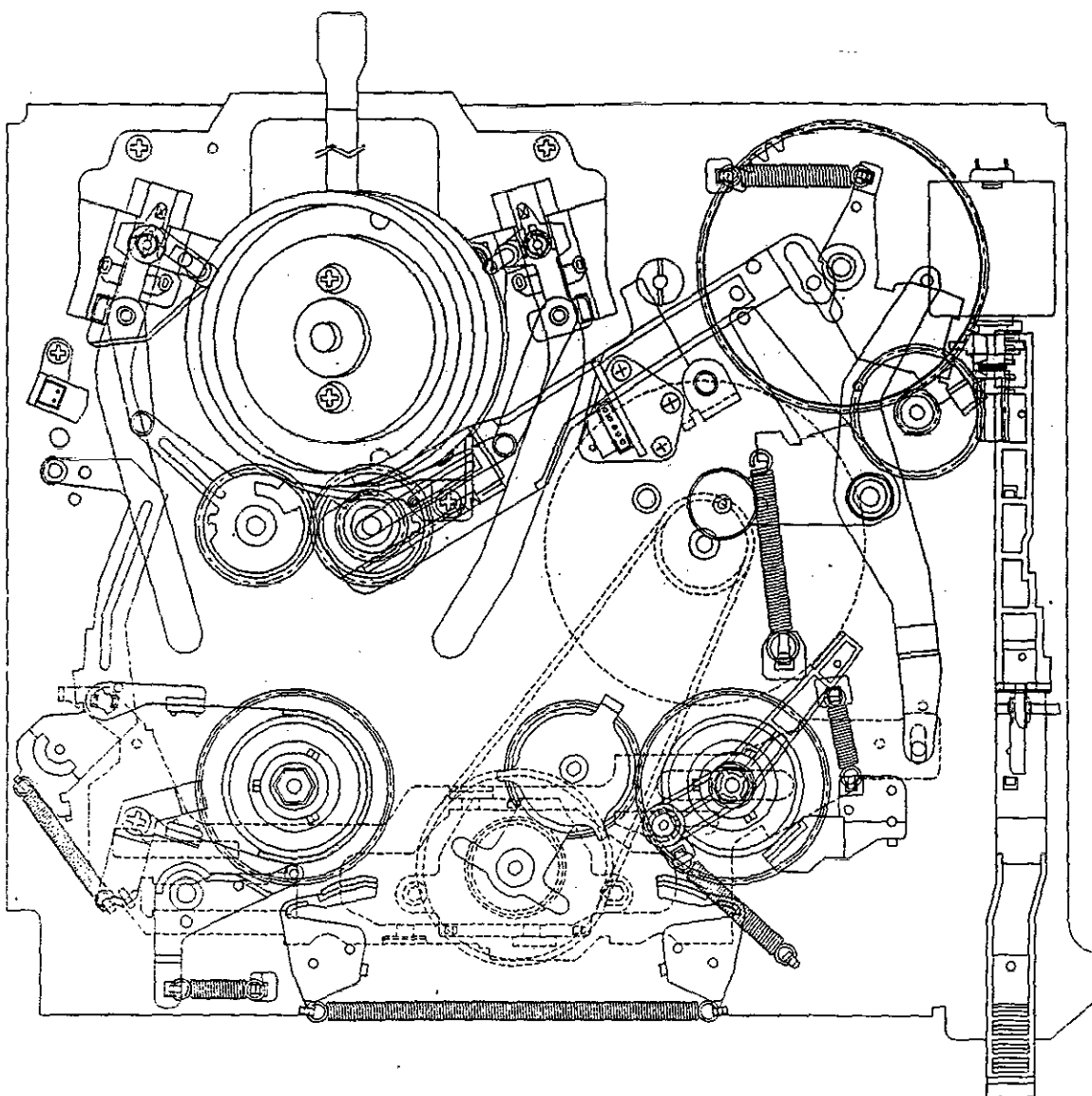
Fig. 1-7. SLOW MODE
