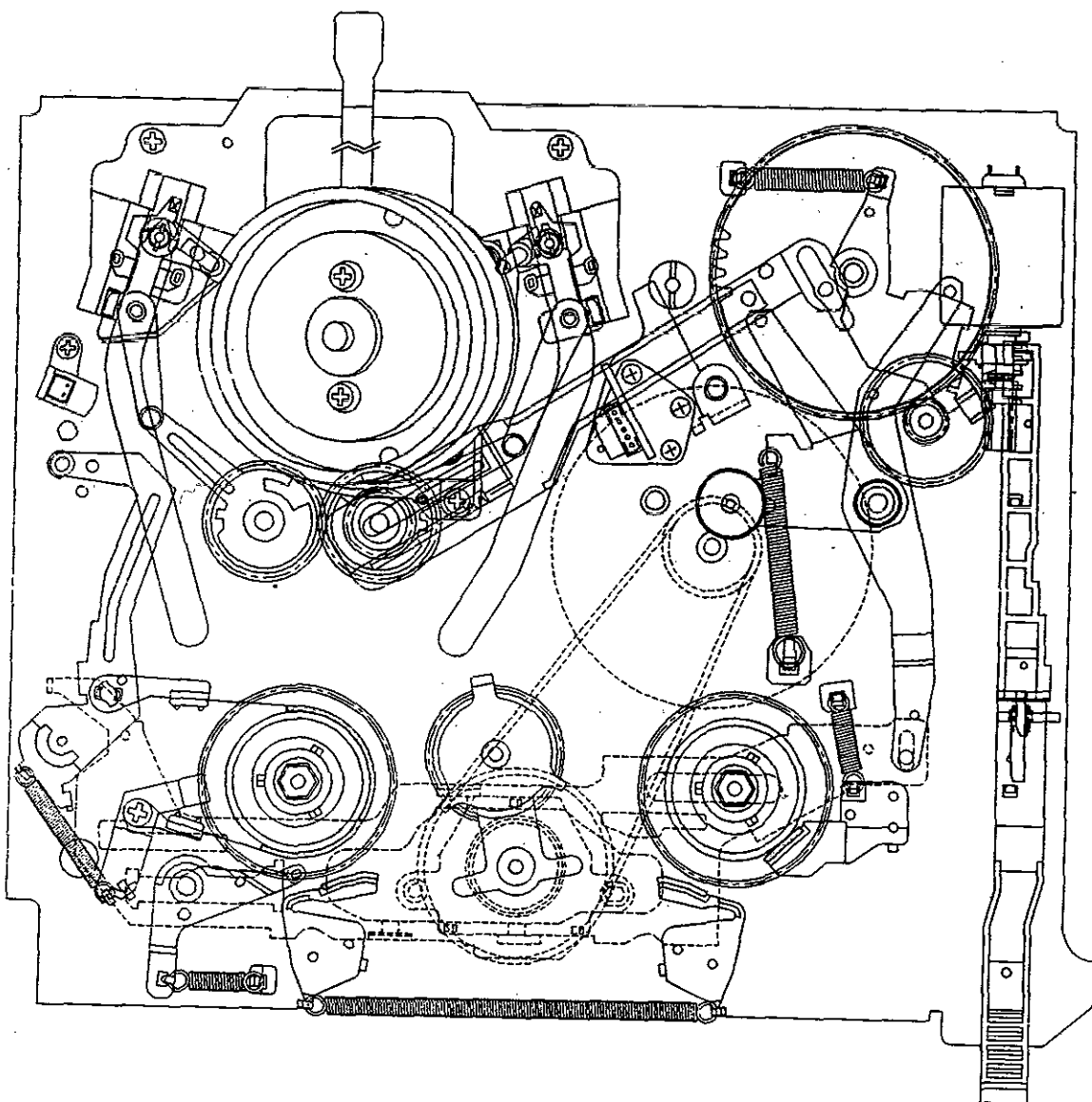
Fig. 1-5. STOP MODE
