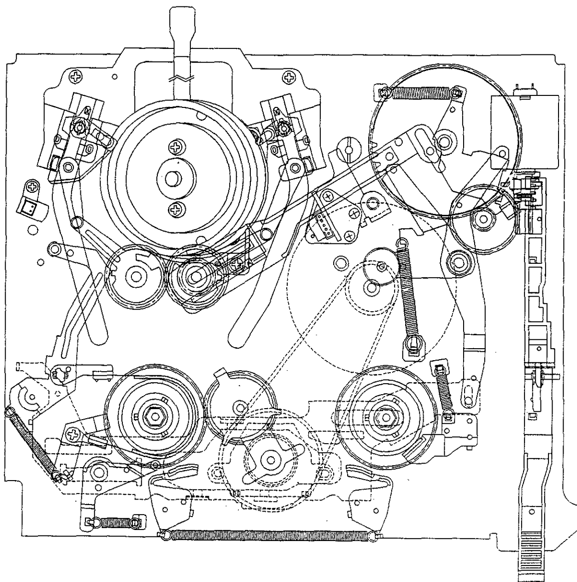
Fig. 1-4. REVIEW MODE
