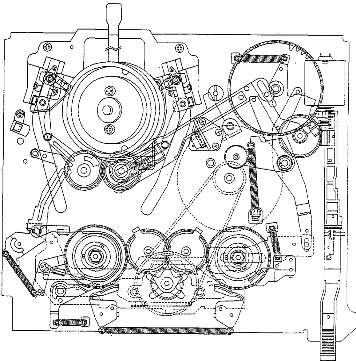
Fig. 1-8. BRAKE MODE
