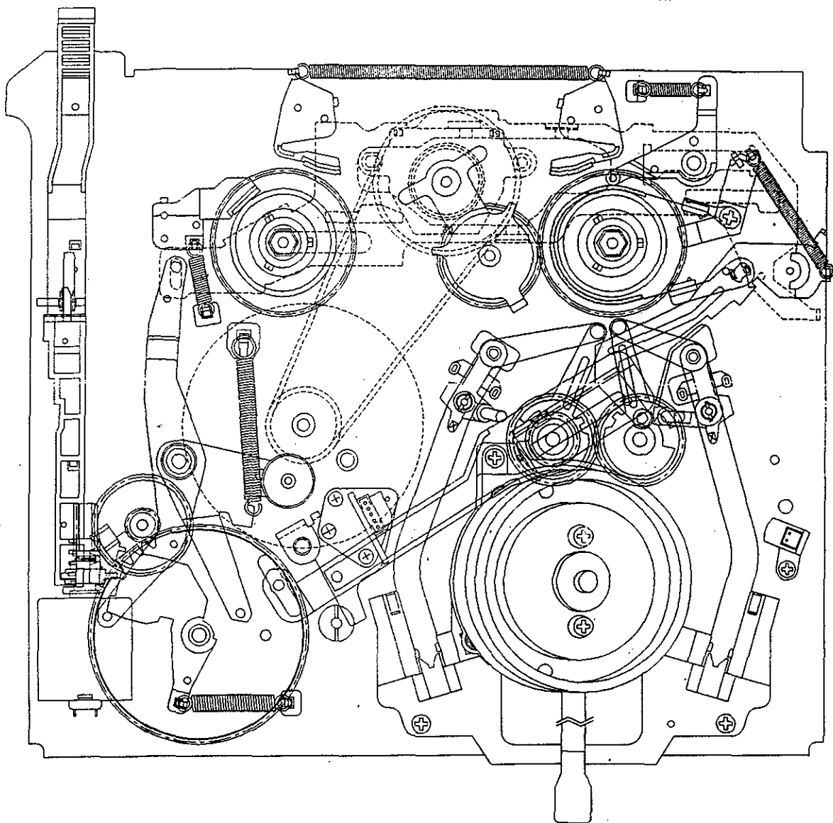
Fig. 1-2. INITIAL MODE
