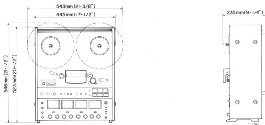
Fig. 2-1 Dimensions
