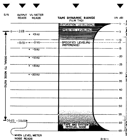
Fig. 7-10 Signal/Noise Computation
