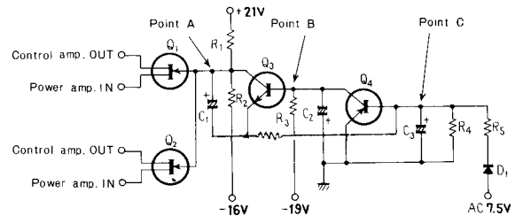
Fig. 5 AF Muting
