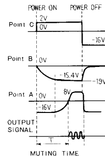
Fig. 5 AF Muting
