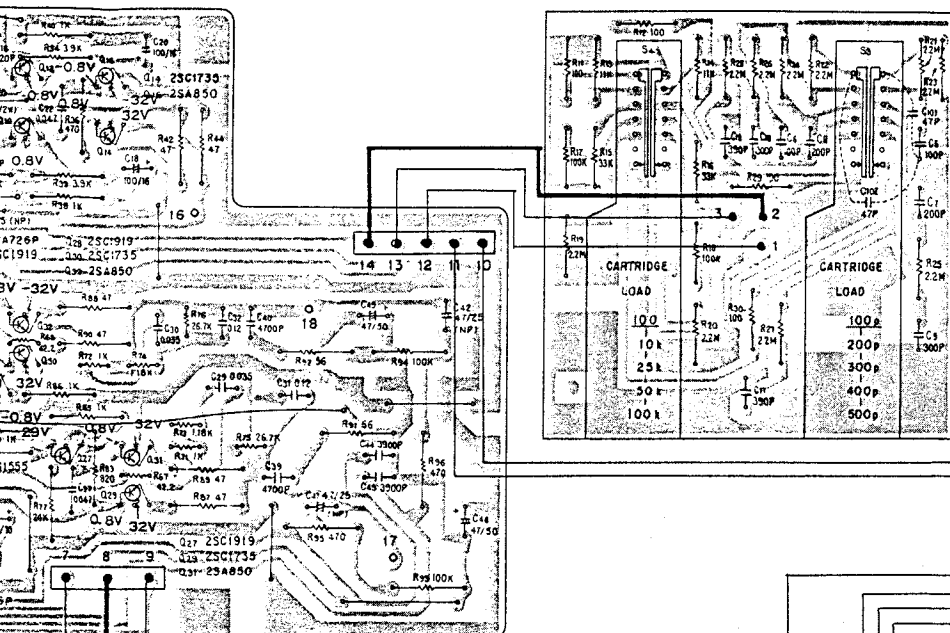
CR ASS'Y (GWX-257)
