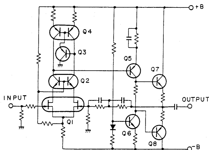
Fig. 5-3 EQ Amplifier
