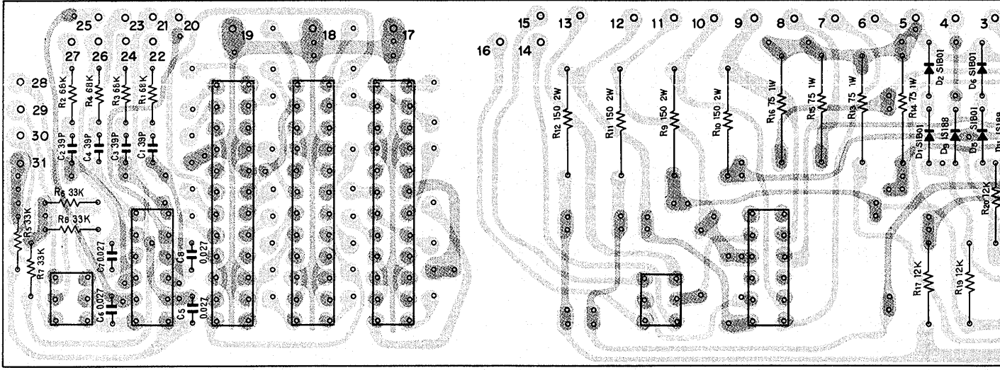
Foil side (AWS-049-A)
