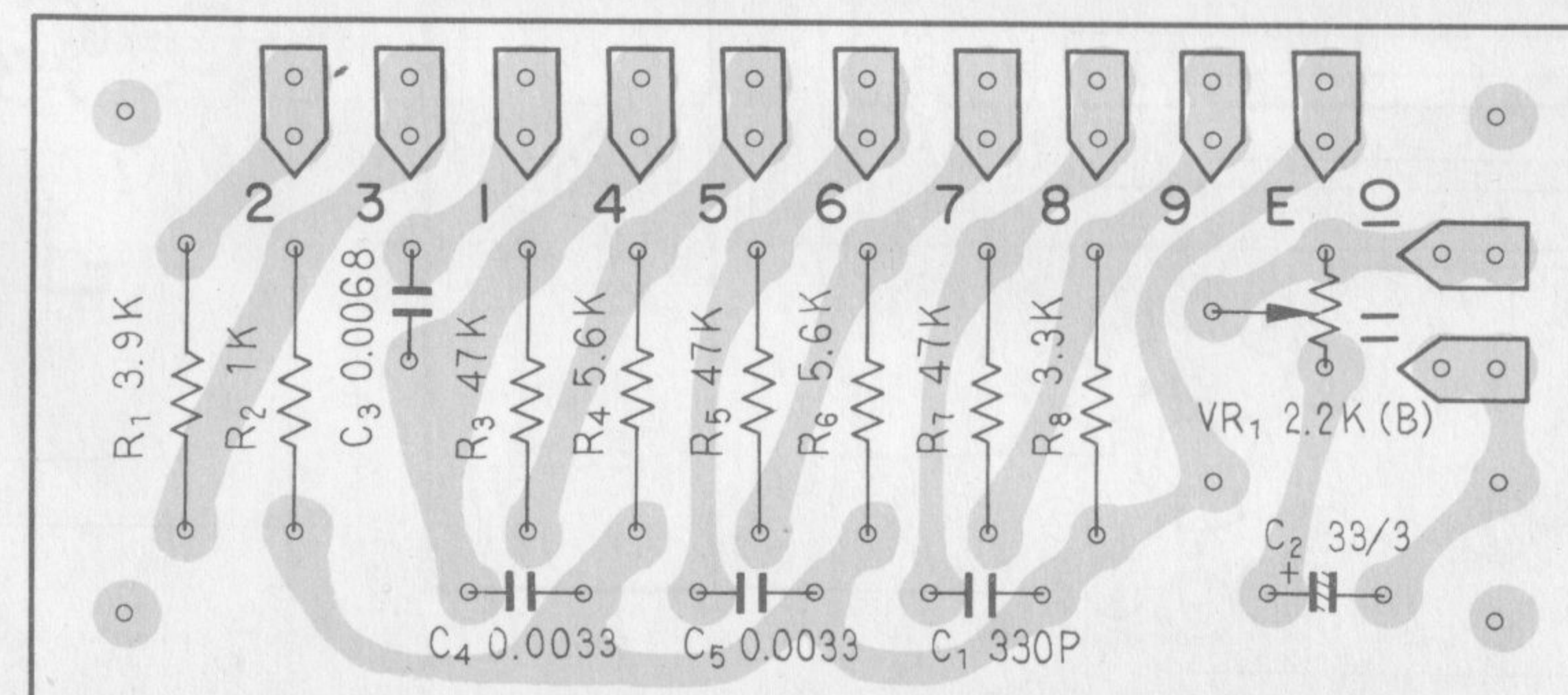
CR ass'y AWE-012 (KUW model)
