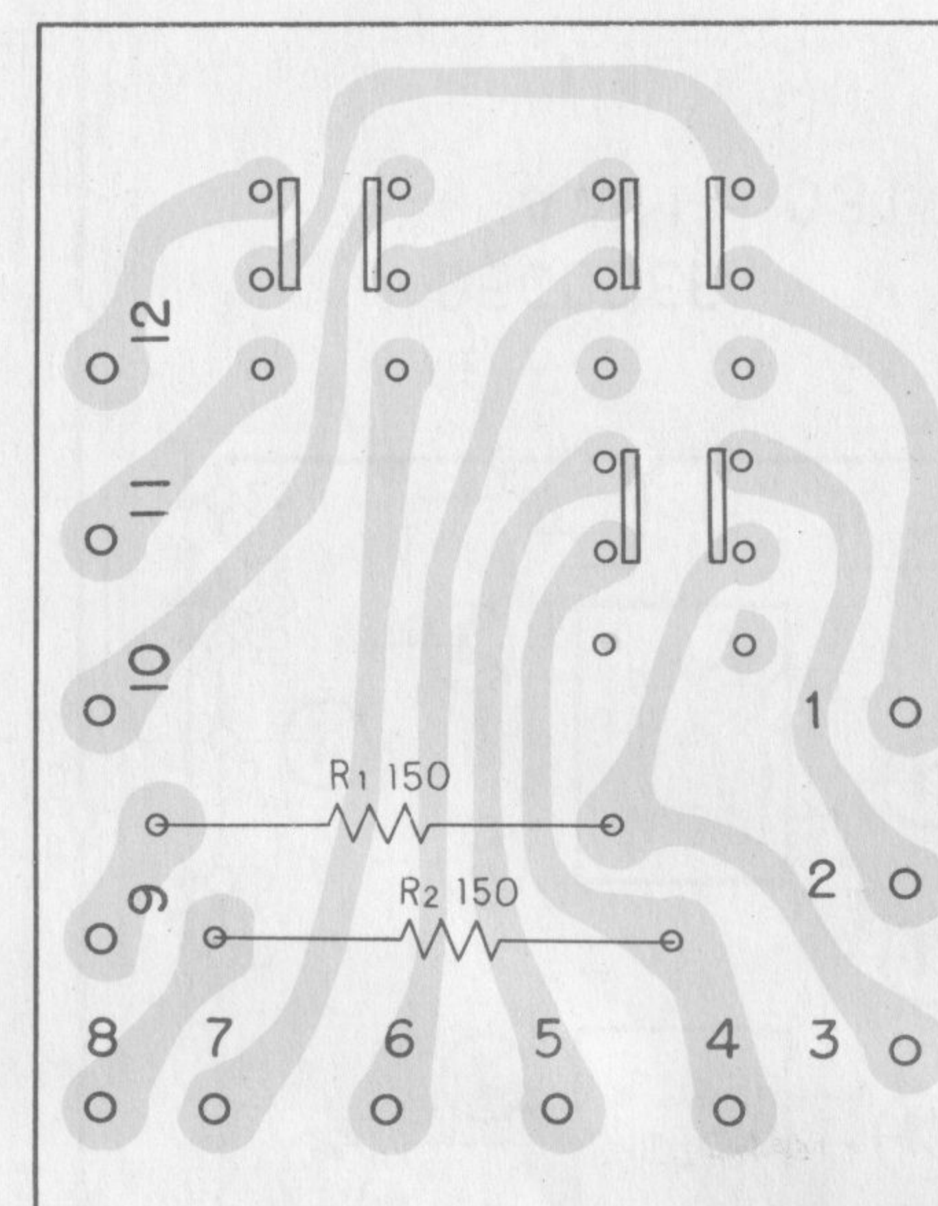
CR ass'y AWE-012 (KUW model)
