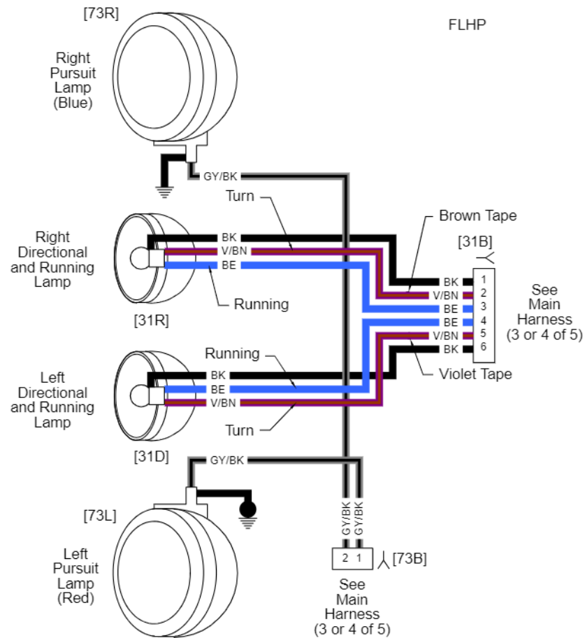
Lighting: 2012 FLHTP, FLHP
