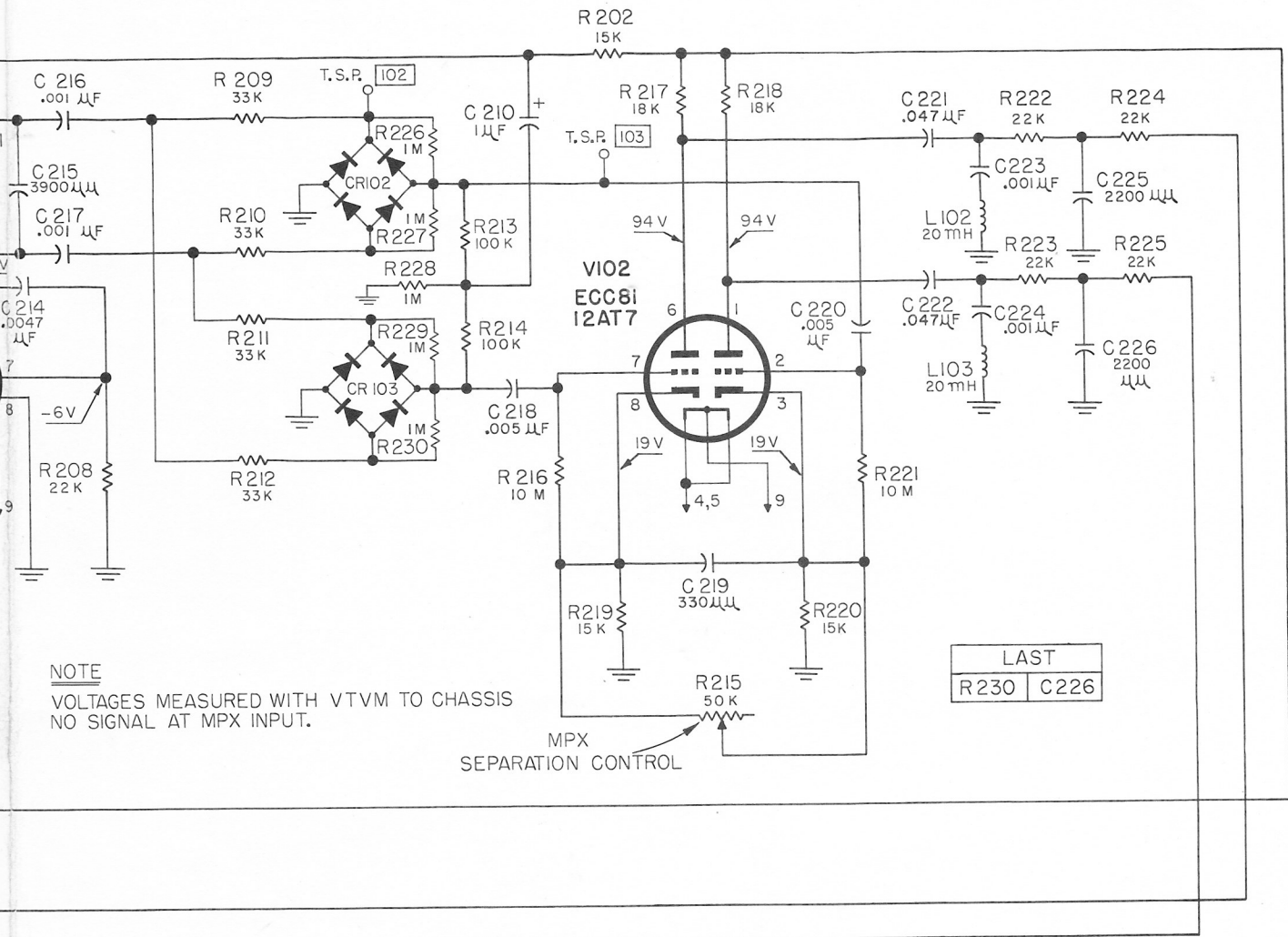
AW#1957B P926WX SCHEMATIC
